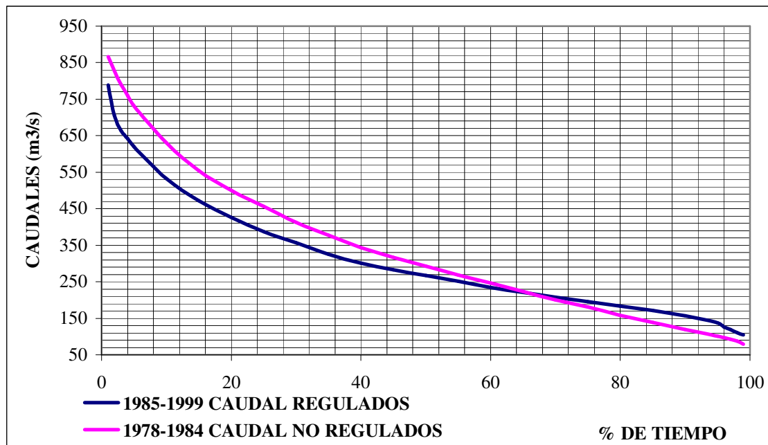
Figura 6.2 Plan de manejo integral de la madre vieja Gota E' Leche CURVA DE DURACION DE CAUDALES DIARIOS - LG MEDIACANOA
